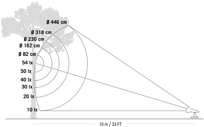
LUX /DISTANCE pour une implantation à 10 m LUX /DISTANCE form a position 33 FT away
