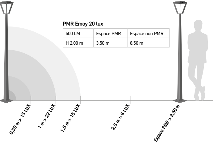
IMPLANTATION LUX /DISTANCE TEST RÉALISÉ AVEC UN LAMPADAIRE TINK551 500 LM
