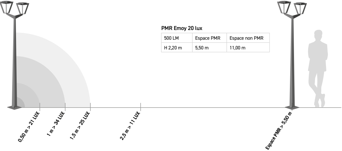
IMPLANTATION LUX /DISTANCE TEST RÉALISÉ AVEC UN LAMPADAIRE TINK555 500 LM
